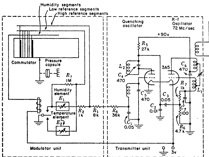
Fig. 10-11.—Radiosonde, AN/AMT-1.
