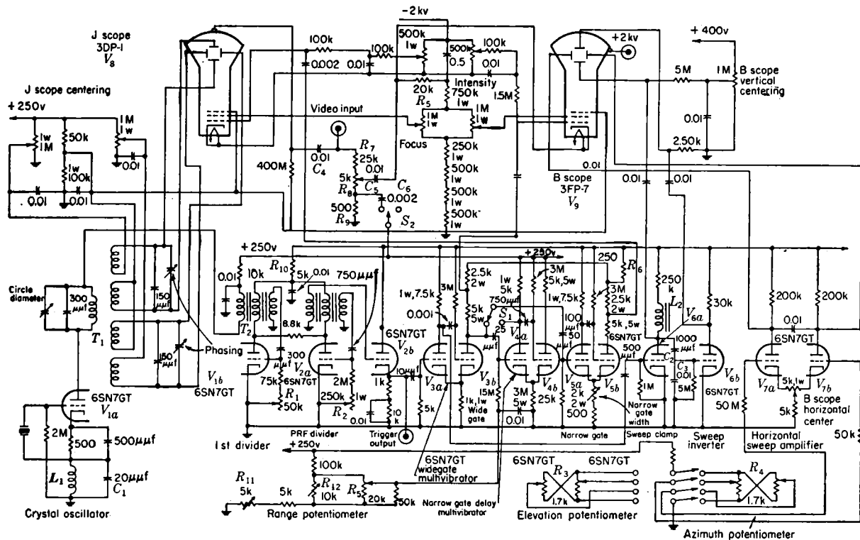
FIG. 7-44.—HR indicator.
